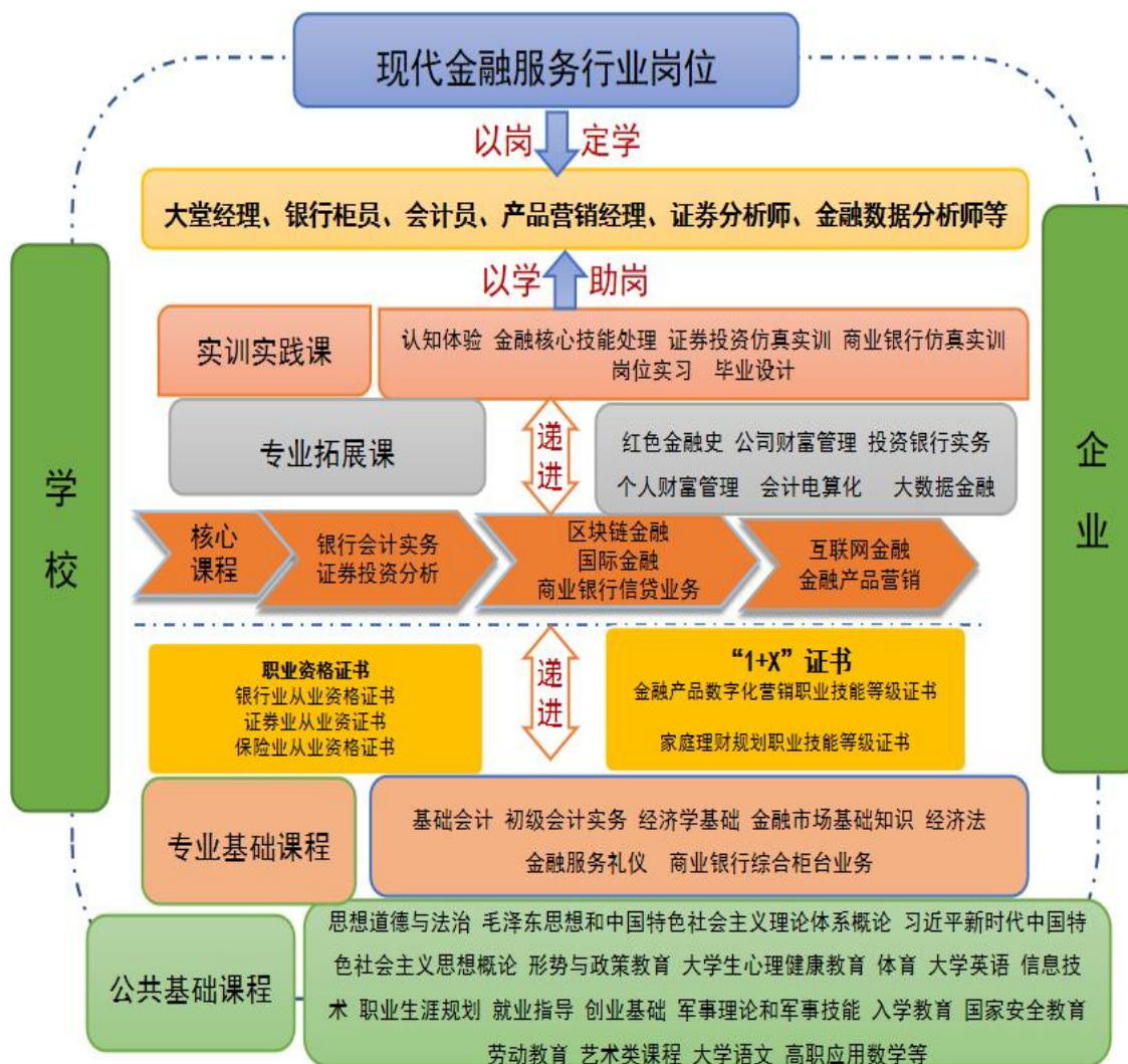
图1 金融服务与管理专业课程体系逻辑图
