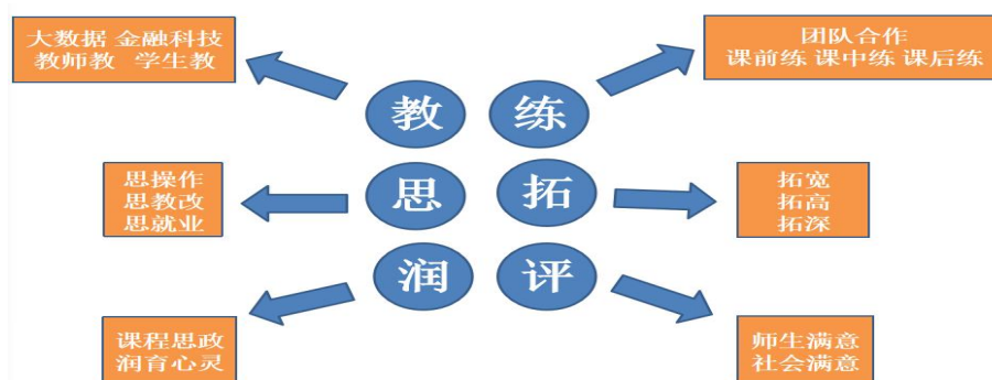
图2 金融服务与管理专业“教练思拓润评”教学模式
